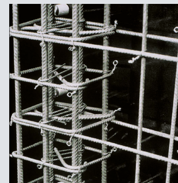
Armature d'une paroi parasismique en béton armé – les détails constructifs et la qualité de l'exécution jouent un rôle crucial dans le comportement des ouvrages soumis à un séisme.
